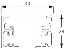
SG 11863 Profil
