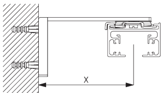
Smart Fix SG 11202 - SG 11204 und Spanner SG 3044: Benötigt Schraube SG 10395 (M4x6).
