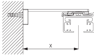
Square Smart Fix SG 11212 - SG 11214 und Spanner SG 3044: Benötigt Schraube SG 10395 (M4x6).
