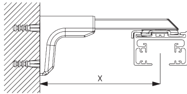
Universal Smart Fix SG 11154 - SG 11156 und Spanner SG 3044: Benötigt Schraube SG 10492 (M4x8).
