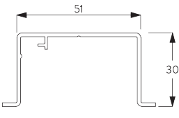
SG 11866 Nutprofil
