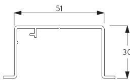
SG 11866 Nutprofil
