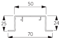
SG 2615 Nutprofil
