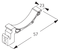
SG 2384 Drahthalter Seitenverspannung
