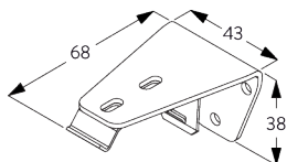
SG 2363 Träger 68 mm
