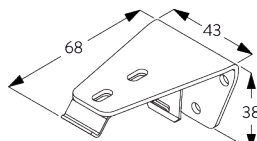
SG 2363 Träger 68 mm
