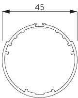
SG 2372 Rohr ø 45mm
