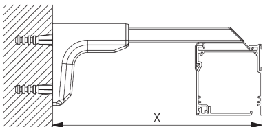
Universal Smart Fix SG 11154 - SG 11156 und Träger SG 2521: Benötigt Schraube SG 10492 (M4x8).
