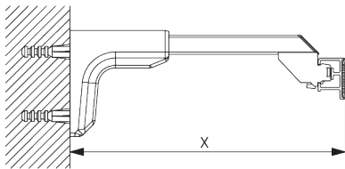
Universal Smart Fix 11154-11156 and Träger SG 3603: Benötigt Schraube SG 10277 (M4x12).
