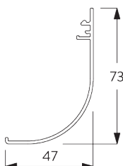
SG 11431 Fascia rond 73 mm
