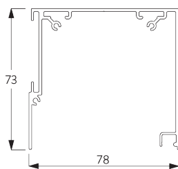
SG 11433 Boîtier 73 mm
