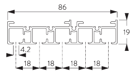
SG 10125 Profil 5-läufig
