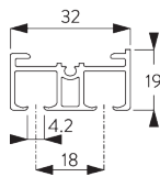
SG 10122 Profil 2-läufig
