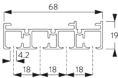
SG 10124 Profil 4-läufig
