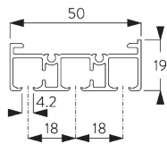
SG 10123 Profil 3-läufig
