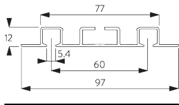
SG 6244p Profil
