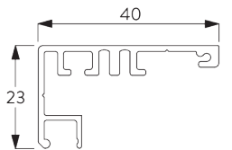
SG 11418 Profil de guidage
